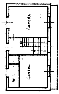
PIANO PRIMO
